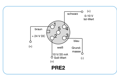
Anschlussplan
